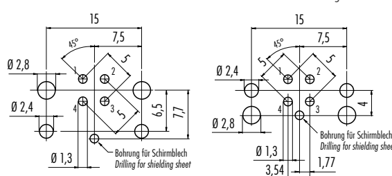
Bohrbilder Buchseneinsatz (Leiterplatte), zweiteilig, mit Schirmblech Drilling schemes female insert (PCB), two-part design, with shielding sheet
