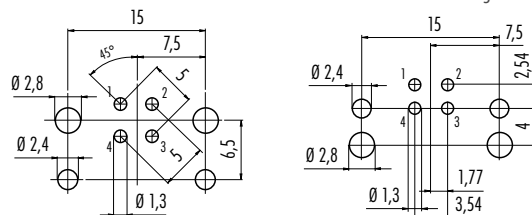
Bohrbilder Buchseneinsatz (Leiterplatte), zweiteilig, ohne Schirmblech Drilling schemes female insert (PCB), two-part design, without shielding sheet
