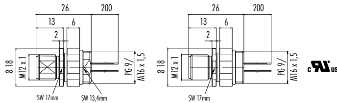
Ausführung mit Zink Druckgussgehäuse Version with zinc diecast housing
