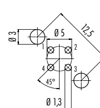
Bohrbilder Buchseneinsatz (Leiterplatte), Metallversion, mit Schirmblech Drilling schemes female insert (PCB), with shielding sheet
