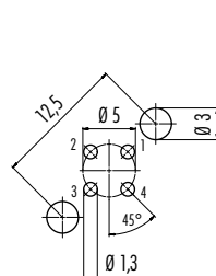
Bohrbilder Stifteinsatz (Leiterplatte), Metallversion, mit Schirmblech Drilling schemes male insert (PCB), metal version, with shielding sheet
